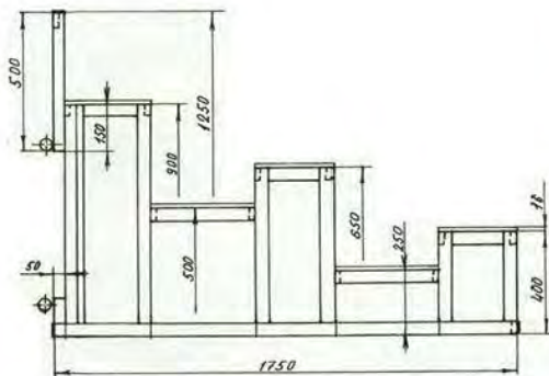
5056 Скамья для раздевалок Тип-1
