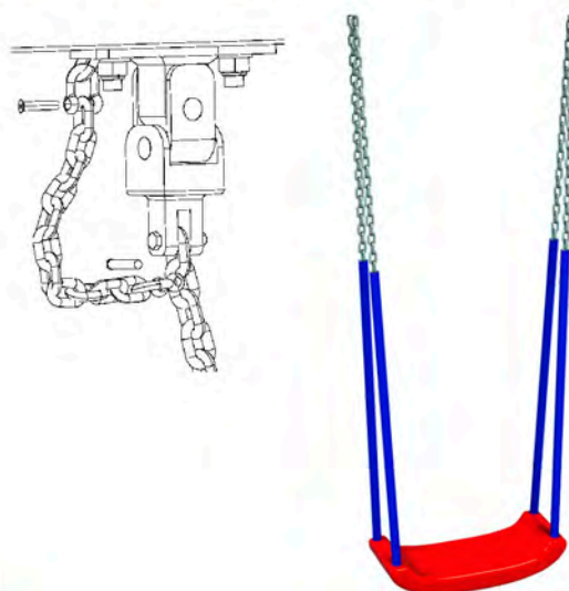
Двойная система крепления цепи к перекладине
